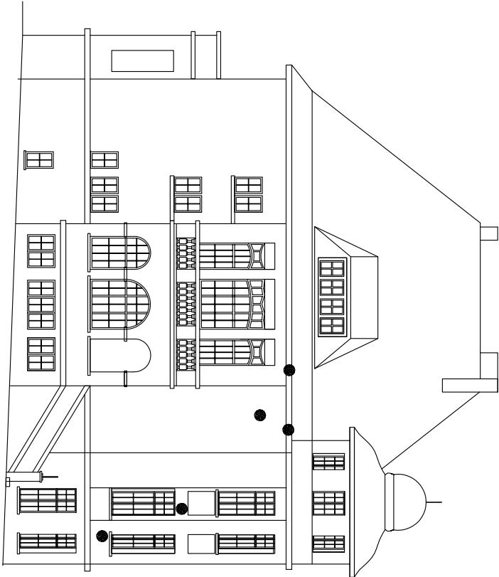
ELEWACJA PÓŁNOCNA
