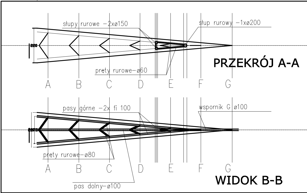
PRZĘKROJE
