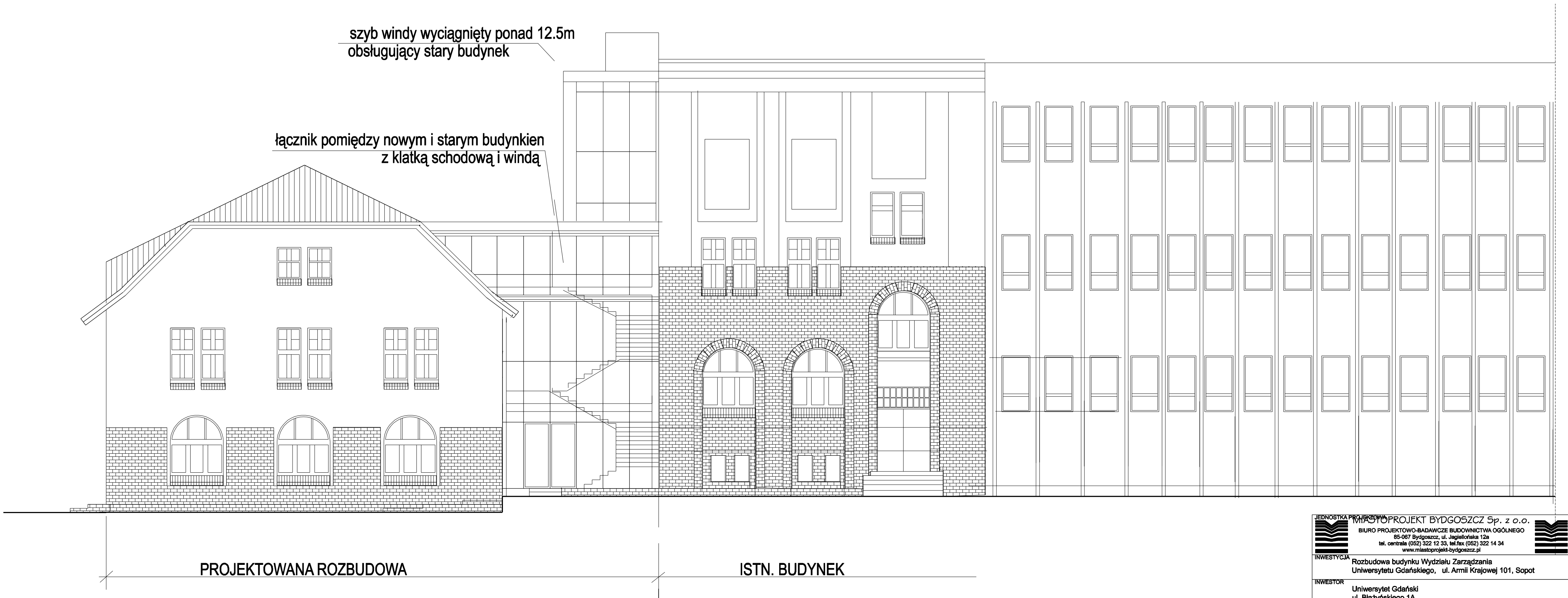
ELEWACJA BOCZNA - ZACHODNIA
